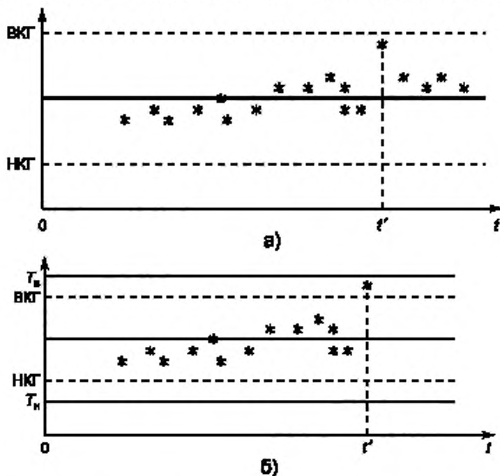
T_n, T_v — нижнее и верхнее предельные значения поля допуска; НКГ, ВКГ — нижняя и верхняя контрольные границы; t' — фиксированный момент времени
