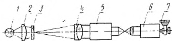
1—источник света; 2—конденсор; 3—миры; 4—объектив коллиматора; 5—анаморфотный киносъёмочный блок или насадка с объективом; 6—микроскоп; 7—окулярный микрометр
