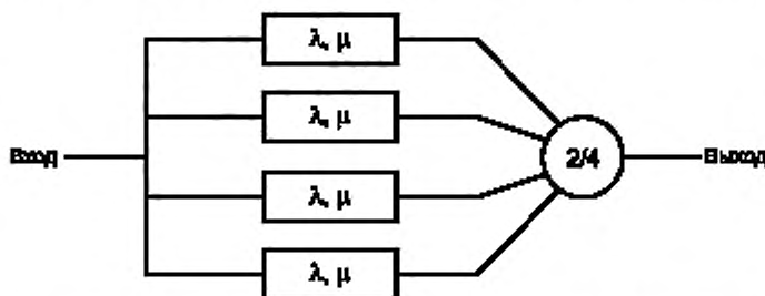
Рисунок 13 — Структурная схема надежности параллельной системы 2/4
