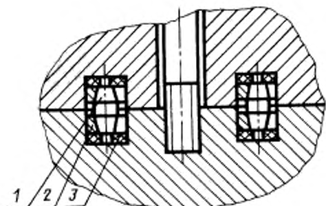
1 — фиксирующий палец; 2 — втулка разрезная; 3 — шайба упругая
