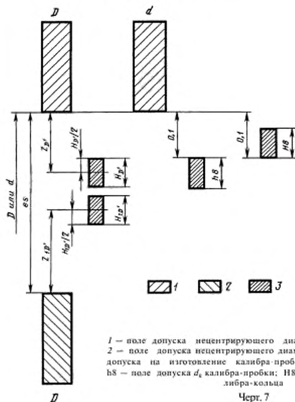
Нецентрирующий диаметр
