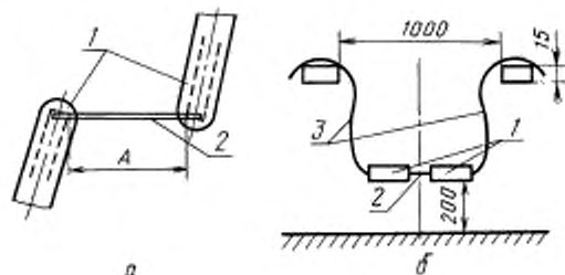
1 — электрододержатель; 2 — стержень; 3 — сварочный кабель
