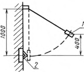
1 — электрододержатель; 2 — уголок
