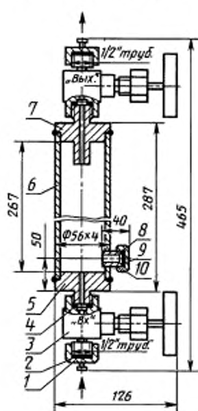
Пробоотборник ПГО-400
