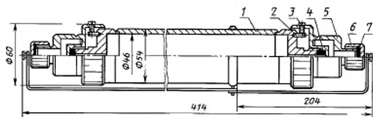
Пробоотборник ПУ-50
