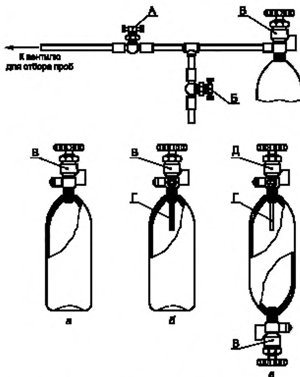
а — контейнер с одним вентиляем; б — контейнер со сливной трубкой; в — контейнер с двумя вентилями; А — регулирующий вентиль; Б — продувочный вентиль; В — впускной вентиль; Г — сливная трубка; Д — выпускной вентиль
