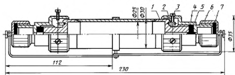
Пробоотборник ПУ-50
