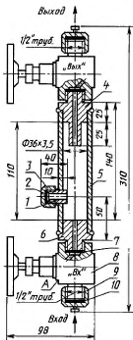
Пробоотборник ПГО-50
