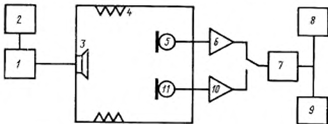
1—генератор; 2—частотомер; 3—громкоговоритель; 4—заглушенная камера; 5 и 11—образцовый и поверяемый микрофоны; 6 и 10—микрофонные усилители; 7—магазин затухания; 8—электронный вольтметр; 9—осциллограф.
