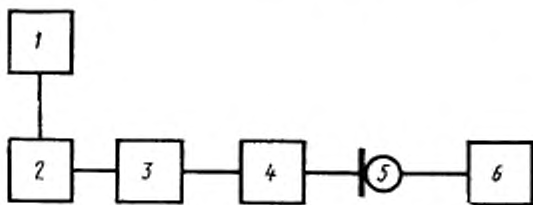
1—частотомер; 2—генератор; 3—магазин затухания; 4—электростатический возбудитель; 5—поворачиваемый микрофон; 6—электронный вольтметр.
