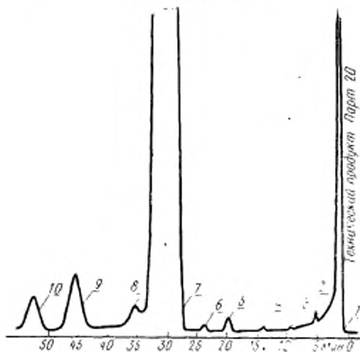
Типовая хроматограмма
