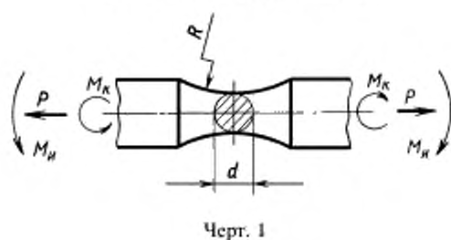
Рабочая часть образца типа I
