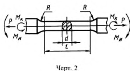
Рабочая часть образца типа II
