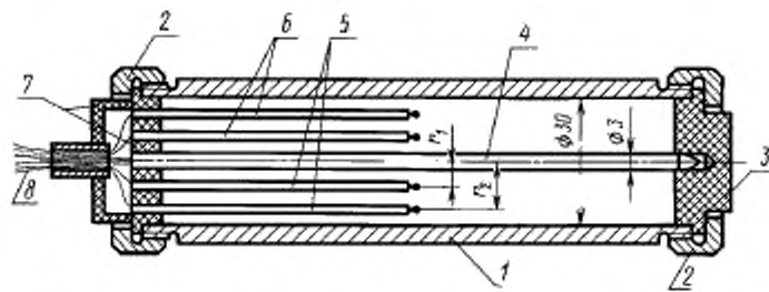
1 — корпус; 2 — накладная гайка; 3 — крышка; 4 — нагреватель; 5, 6 — термометры; 7 — крышка. y — выходы термометр и нагревателя
