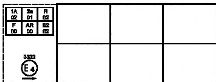
Рисунок 2 — Упрощенная маркировка для сгруппированных, комбинированных или совмещенных огней
