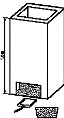
Рисунок 10 — Корзина, контейнер и стружка
