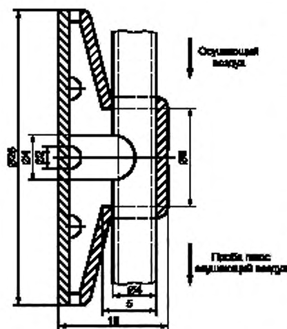
Рисунок 9 — Пробоотборник
