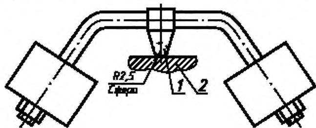
1 — стальной шарик диаметром 5 мм; 2 — образец
