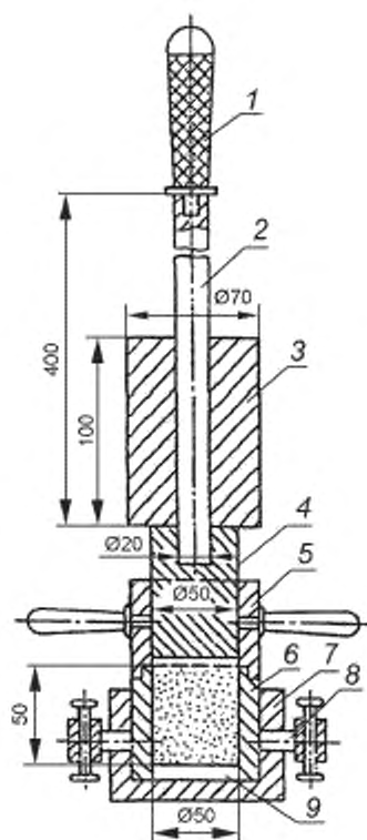
1 — рукоятка; 2 — направляющий стержень; 3 — гиря; 4 — плунжер; 5 — направляющий насадный цилиндр. 6 — разъемный цилиндр; 7 — подотканник; 8 — закрепляющие винты; 9 — металлическая пластинка
