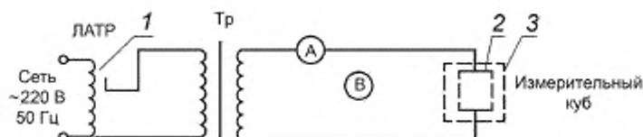
1 — лабораторный регулировочный трансформатор (ЛАТР). 2 — электрод 3 — измерительный куб
