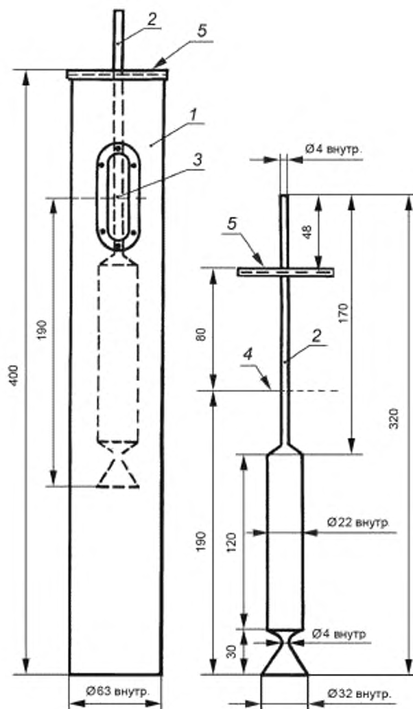
Рисунок 2 — Металлический цилиндр и мерная пипетка
