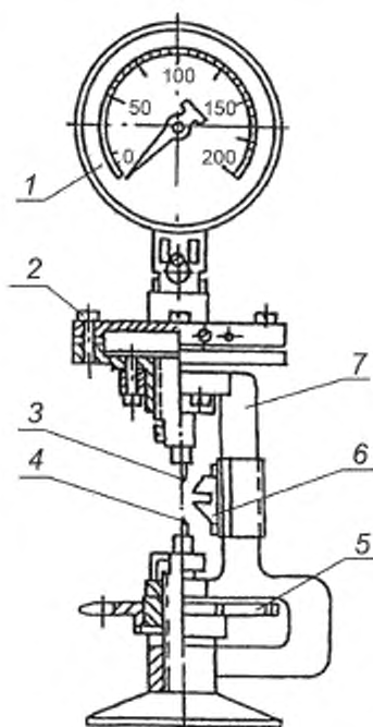
1 — манометр; 2 — гидравлическая мерсдоза; 3 — верхний зуб; 4 — нижний зуб; 5 — диск винтового механизма; 6 — щелевой упор; 7 — корпус прибора
