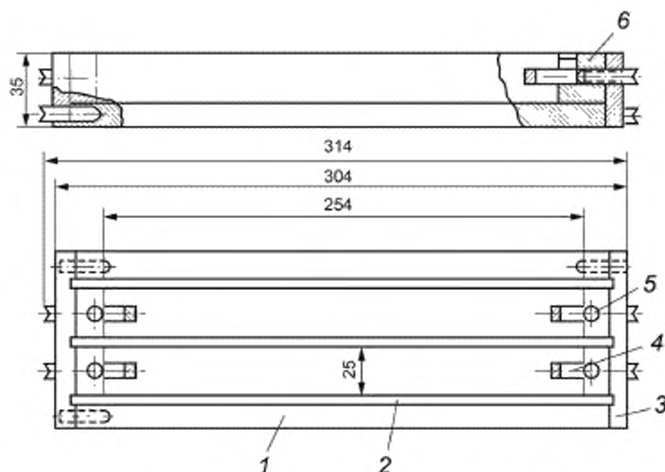
1 — форма; 2 — боковые стенки формы; 3 — торцевая стенка формы; 4 — репер; 5 — столорный винт для крепления репера, 6 — держатель репера
