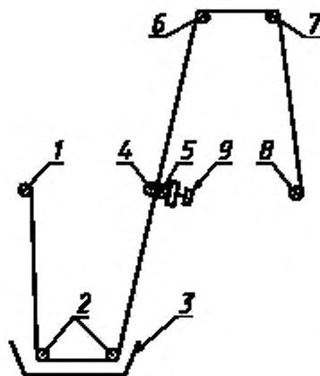
1 — катушка для намотки ткани; 2 — загрязняющая ванна; 3 — направляющие ролики; 4, 5 — обжимные ролики; 6, 7 — направляющие ролики; 8 — приемная катушка; 9 — прижимное устройство
