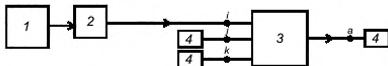
1 — панорамный измеритель КСВН; 2 — рефлектометр на проверяемую полосу частот; 3 — устройство сложения; 4 — согласованные нагрузки; i, j, k — входы устройства сложения
