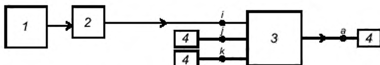
1 — измеритель комплексных сопротивлений; 2 — коаксиальный переход; 3 — устройство сложения; 4 — согласованные нагрузки; i, j, k — входы устройства сложения
