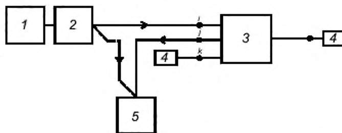
1 — измерительный генератор; 2 — развязывающий аттенюатор; 3 — устройство сложения; 4 — согласованные нагрузки; 5 — измеритель высокочастотного (ВЧ) напряжения; i, j, k — входы устройства сложения
