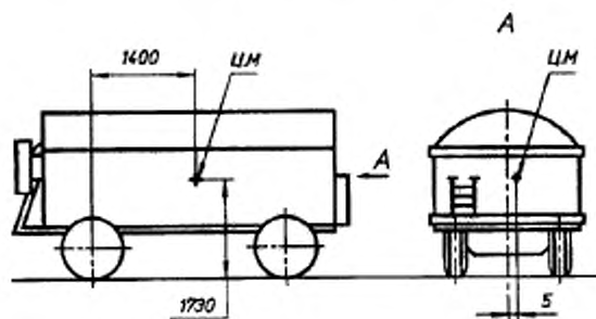
Рисунок 1 — Центр массы электростанции
