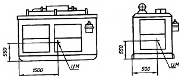
Рисунок 2 — Центр массы электроагрегата
