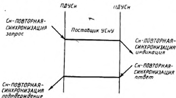
Рисунок 15 — Последовательность примитивов услуги Сн-ПОВТОРНАЯ-СИНХРОНИЗАЦИЯ
