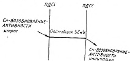
Рисунок 19 — Последовательность примитивов услуги ВОЗОБНОВЛЕНИЕ-АКТИВНОСТИ
