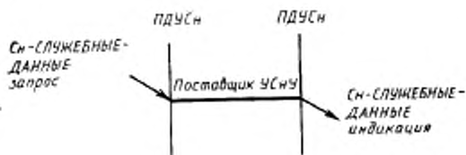
Рисунок 8 — Последовательность примитивов услуги Сн-СЛУЖЕБНЫЕ-ДААННЫЕ
