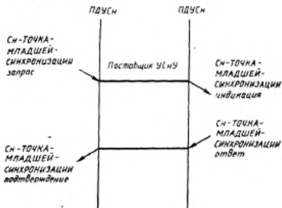
Рисунок 13 — Последовательность примитивов услуги Сн-ТОЧКА-МЛАДШЕЙ-СИНХРОНИЗАЦИИ
