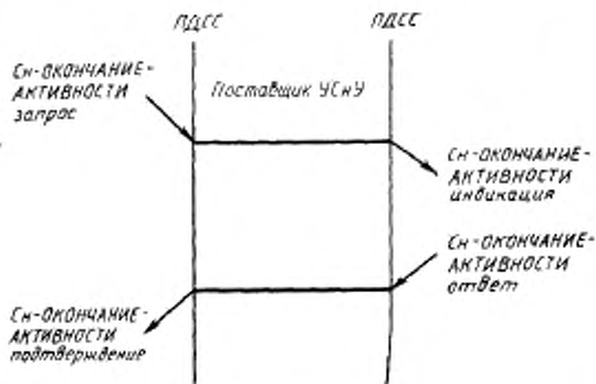
Рисунок 22 — Последовательность примитивов услуги Cn-OKONCHANIJE-AKTIVNOSTI
