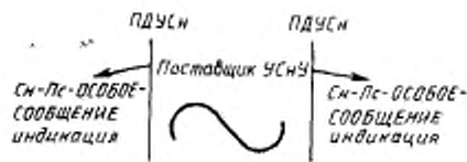
Рисунок 16 — Последовательность примитивов услуги Сн-Пс-ОСОБОЕ-СООБЩЕНИЕ
