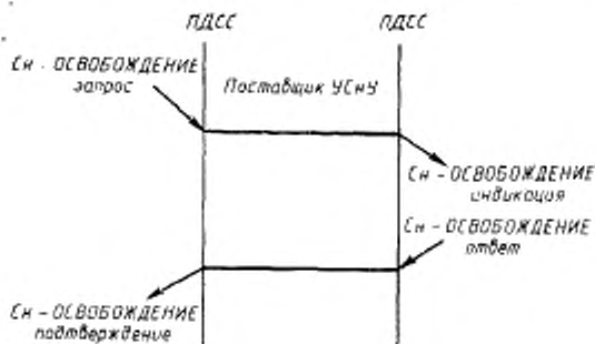
Рисунок 23 — Последовательность примитивов услуги Сл-ОСВОБОЖДЕНИЕ
