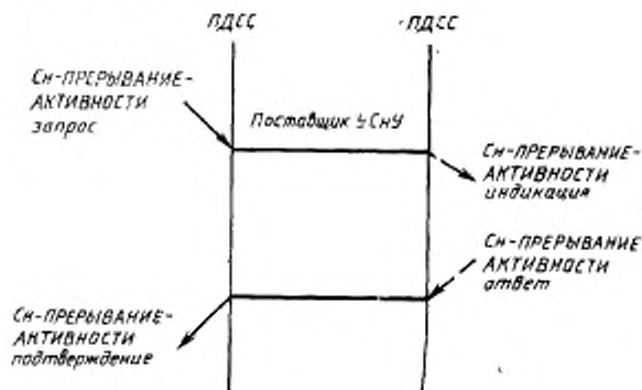
Рисунок 20 — Последовательность примитивов услуги Сл-ПРЕРЫВАНИЕ-АКТИВНОСТИ
