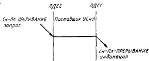
Рисунок 24 — Последовательность примитивов услуги Сл-Пл-ПРЕРЫВАНИЕ
