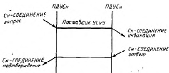
Рисунок 5 — Последовательность примитивов услуги Сн-СОЕДИНЕНИЕ
