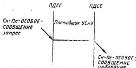
Рисунок 17 — Последовательность примитивов услуги Ся-Пл-ОСОБОЕ-СООБЩЕНИЕ
