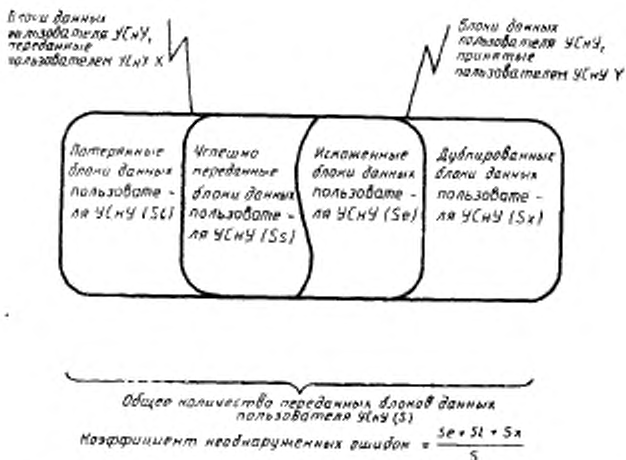
Рисунок 4 — Компоненты коэффициента недобнаруженных ошибок
