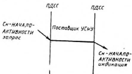
Рисунок 18 — Последовательность примитивов услуги НАЧАЛО-АКТИВНОСТИ
