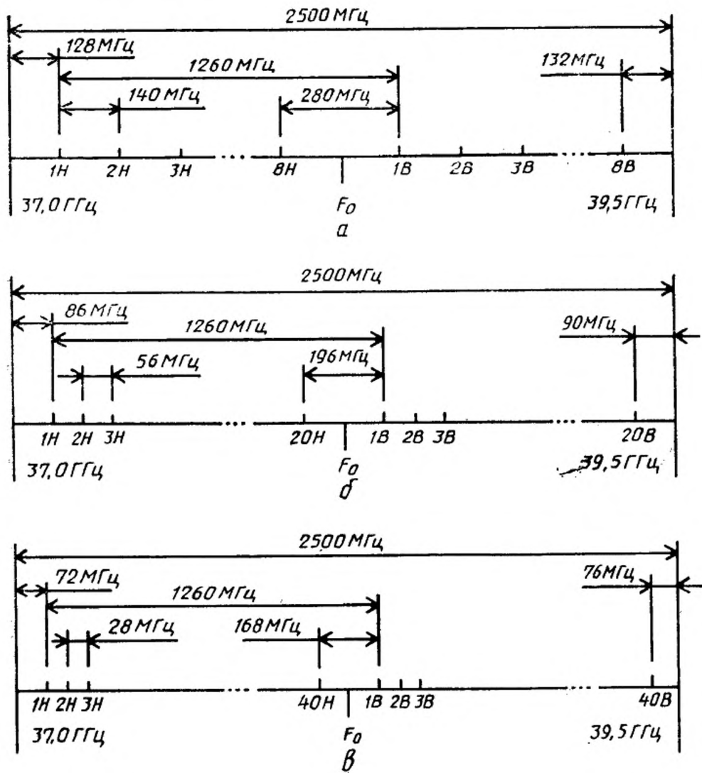
Рисунок Б.17 — Частотный план радиорелейной системы, работающей в диапазоне 37,0—39,5 ГГц: а) разнос между фиксированными частотами 140 МГц; б) разнос между фиксированными частотами 56 МГц; в) разнос между фиксированными частотами 28 МГц.
