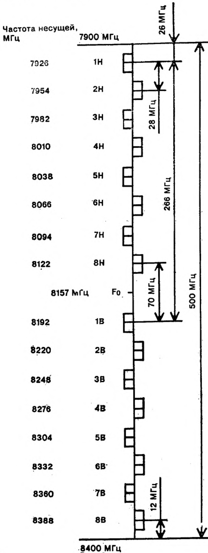
Рисунок Б.7. — Частотный план радиорелейной системы, работающей в диапазоне 8 ГГц
