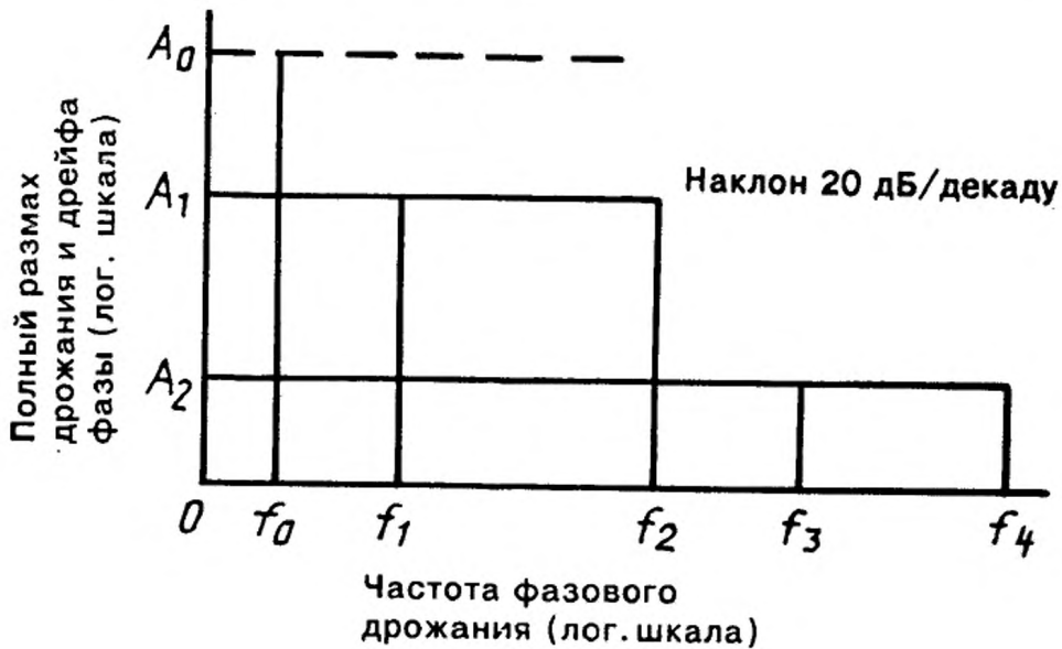
Рисунок 11 — Шаблон максимального допустимого входного фазового дрожания и дрейфа фазы для аппаратуры радиорелейных систем плездохронной цифровой иерархии
