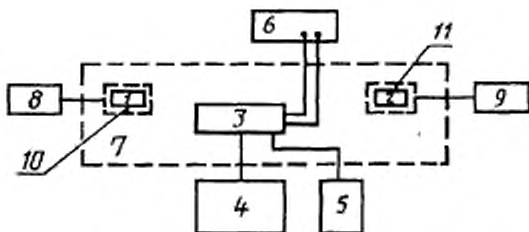
1 — излучатель опорного лазера; 2 — излучатель исследуемого лазера; 3 — оптический блок; 4 — измерительный блок; 5 — баллон с газом (сжатые гелий или азот); 6 — осциллограф; 7 — общее основание; 8 — блок управления опорного лазера; 9 — блок управления исследуемого лазера; 10, 11 — юстируемые подставки для лазера
