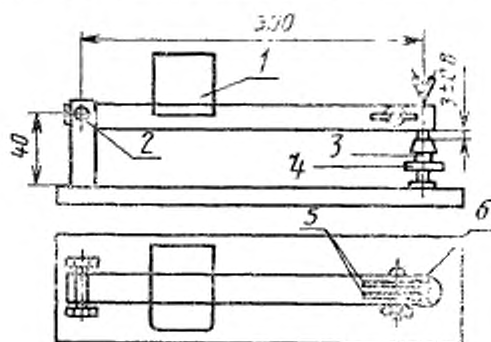
1 — перемещающийся нос; 2 — шарнирный валец; 3 — патрон; 4 — опора для патрона, чтобы рычаг находился в горизонтальном положении, когда усилие прилагают первый раз; 5 — прорези в рычаге для более удобного захвата провода патрона; 6 — отверстия для проводов
