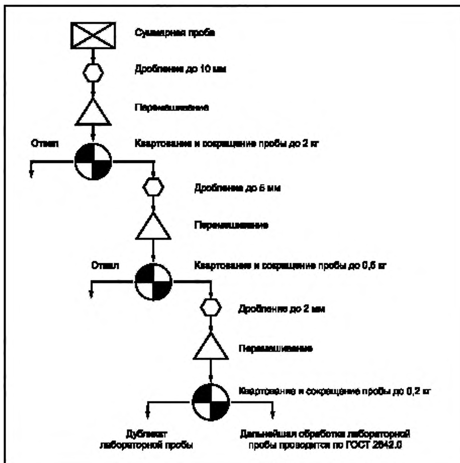
Рисунок В.1 — Схема подготовки проб сыря
