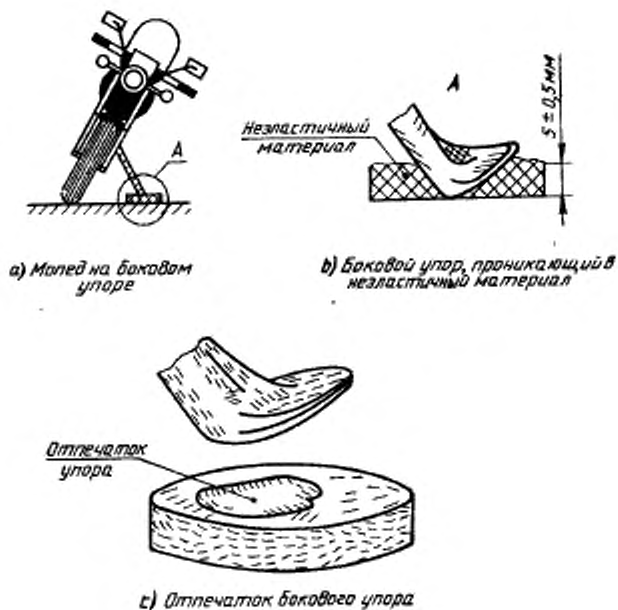
Рисунок 1 — Боковой упор
