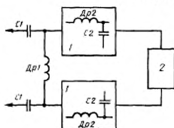
Измерительная схема
