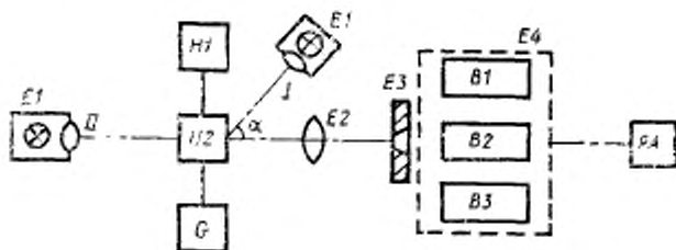
Н1 —контрольный индикатор или светофильтр; Н2 —проверяемый индикатор; Е1 —осветитель (положение 1 —«на отражение»; положение II —«на просвет»); G —источник питания индикатора; Е2 —линза; Е3 —диафрагма фотоэлектрического колориметра; Е4 —фотоэлектрический колориметр; В1 , В2 , В3 —фотоприемники, спектральная чувствительность которых скорректирована к функциям сложения цветов или их линейной комбинации; РА —регистрирующий прибор; \alpha —угол освещения индикатора (в режиме «на отражение» \alpha=(45\pm 5)^\circ\text{C} , в режиме «на просвет» \alpha=(60\pm 5)^\circ\text{C} ).
