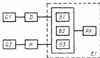
G1 —блок установки электрического режима контрольного источника излучения; D —контрольный источник излучения; G2 —блок установки электрического режима измеряемого индикатора; H —проверяемый индикатор; B1 , B2 , B3 —фотоприемники; PA —регистрирующий прибор; E1 —колориметр
