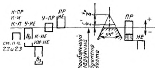
Калибры для контроля болтов (наружной резьбы)
