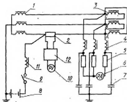
1 — питающий трансформатор; 2 — шунт; 3 — измераемая обмотка; 4 — индуктивность; 5 — резистор; 6 — микроамперметр; 7 — конденсатор; 8 — аккумуляторная батарея; 9 — выключатель; 10 — милливольтметр; 11 — дроссель; 12 — фильтр
