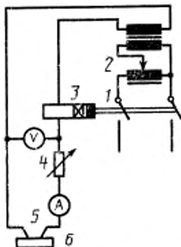
1 — выключатель; 2 — источник переменного тока на 100—600 В; 3 — защитный резистор; 4 — переменный резистор; 5 — электрод; 6 — образец
