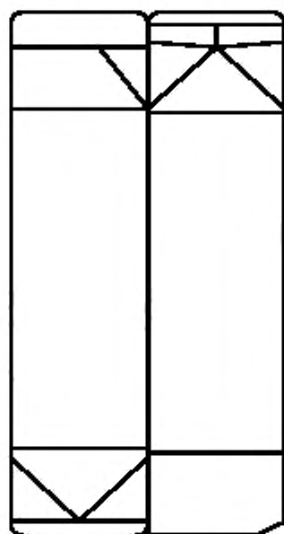
Рисунок А.5 — Заготовка коробки — высе- ка с нанесенными линиями сгиба (биговкой) и продольным сварным швом
