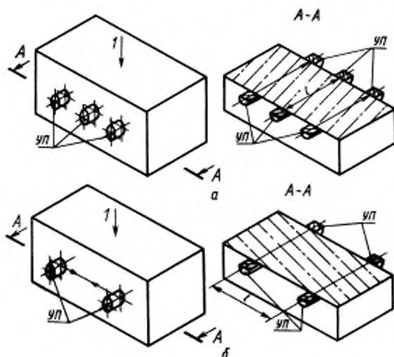
a — схема испытания призм способом сквозного прозвучивания, б — схема испытания призм способом поверхностного прозвучивания; УП — ультразвуковые преобразователи; I — направление формирования
