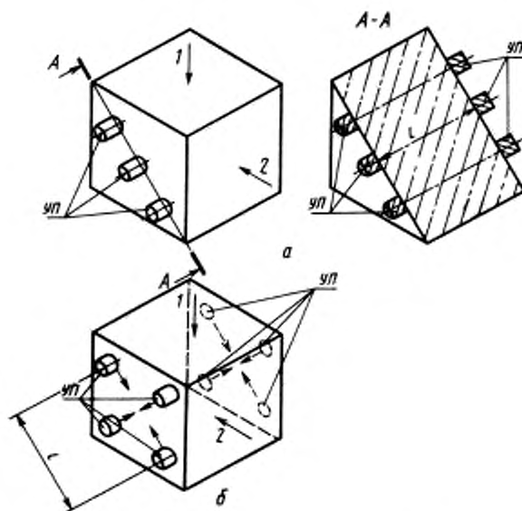
а — схема испытания кубов способом сквозного прозвучивания; б — схема испытания кубов способом поверхностного прозвучивания; УП — ультразвуковые преобразователи; 1 — направление формирования; 2 — направление испытания при сжатии; l — база прозвучивания
