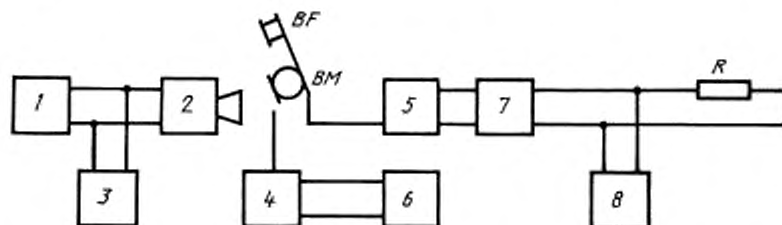
1 — генератор сигналов низкочастотный (генератор шума при измерении амплитудной характеристики); 2 — рот искусственный; 3, 6, 8 — электронные вольтметры переменного напряжения для измерения синусоидального сигнала, для измерения сигнала произвольной формы (при измерении амплитудной характеристики); 4 — зонд акустический; 5 — измеряемый ТА; 7 — питающий комплект; BF — телефон испытуемого ТА; BM — микрофон испытуемого ТА, R — резистор сопротивлением (600 \pm 60) Ом, мощностью не менее 0,25 Вт
