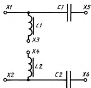
C1, C2 — конденсаторы емкостью (4 \pm 0,2) мкФ; L1, L2 — дроссели с индуктивностью обмотки не менее 2 Гн при токе подмагничивания 60 мА, с активным сопротивлением (500 \pm 50) Ом для напряжения (60 \pm 3) В, с активным сопротивлением (400 \pm 40) Ом для напряжения (48 \pm 2,4) В, X1, X2 — контакты подключения АД; X3, X4 — контакты подключения источника питания; X5, X6 — контакты подключения СЛ
