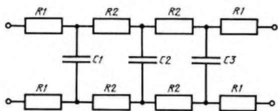
R1 — резистор с сопротивлением (52,5 \pm 0,5) Ом; R2 — резистор с сопротивлением (105 \pm 1) Ом; C1 — C3 — конденсаторы емкостью (55,0 \pm 0,3) нФ
