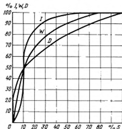
S — разборчивость слогов; W — разборчивость слов; D — разборчивость звуков; I — разборчивость фраз
