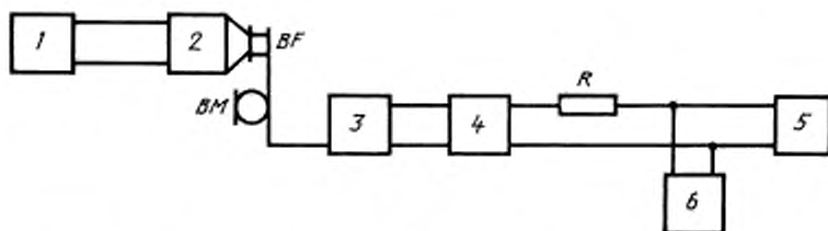
1, 6 — электронные вольтметры переменного напряжения; 2 — ухо искусственное; 3 — испытуемый телефонный аппарат; 4 — питающий комплект; 5 — генератор сигналов низкочастотный; BF — телефон испытуемого ТА; BM — микрофон испытуемого ТА; R — резистор сопротивлением (600 \pm 60) Ом, мощностью не менее 0,25 Вт
