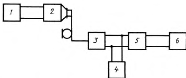
1, 4 — электронные вольтметры переменного напряжения; 2 — ухо искусственное; 3 — измеряемый ТА; 5 — питающий комплект; 6 — генератор сигналов низкочастотный
