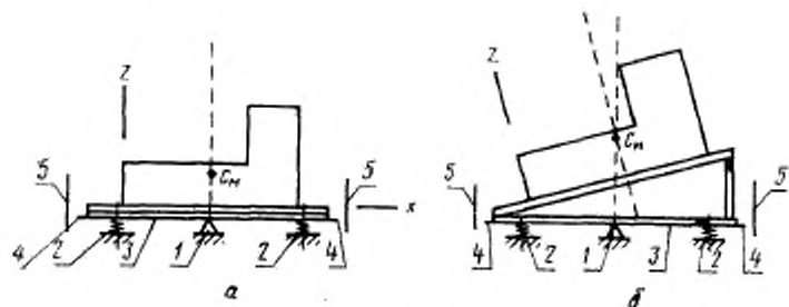
а — определение координат x_c и y_c ; б — определение координаты z_c ; 1 — нож; 2 — нежесткие страховочные упругие опоры; 3 — раздвижная рама; 4 — стрелки указателя уровня; 5 — шкалы; С — центр тяжести машины
