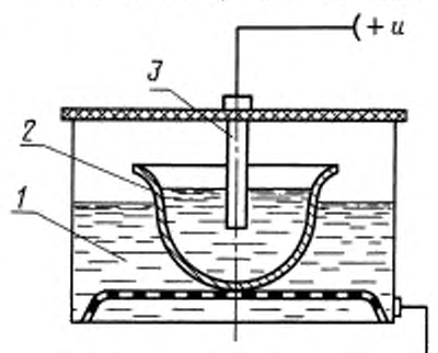
1 — электролит; 2 — корпус каски; 3 — подвижной электрод
