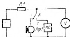
Г—звуковой генератор, R_1 —резистор, сопротивление которого должно превышать модуль полного сопротивления не менее чем в 20 раз; МС—магазин сопротивлений; V—электронный вольтметр; Лрп—ларингофон; B1—переключатель.
