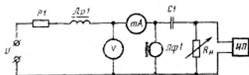
R1 —резистор; Lp1 —дроссель; V —вольтметр постоянного тока; mA —миллиамперметр постоянного тока; C1 —разделительный конденсатор; R n —нагрузочный резистор; ИП —измерительный прибор (вольтметр, измеритель нелинейных искажений, прибор для автоматической записи частотных характеристик); Lf —ларингофон; U —напряжение источника тока
