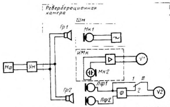
Мф—магнитофон; Ум—усилитель мощности с корректирующим устройством; Гр1 и Гр2—система громкоговорителей; ШМ—шумомер; МК—измерительный микрофон или акустический асд; Лф1 и Лф2—комплект ларингофонов; Ф—фильтры (октавные или третьоктавные); V1 и V2—электронные вольтметры квадратичного типа; В—переключатель.
