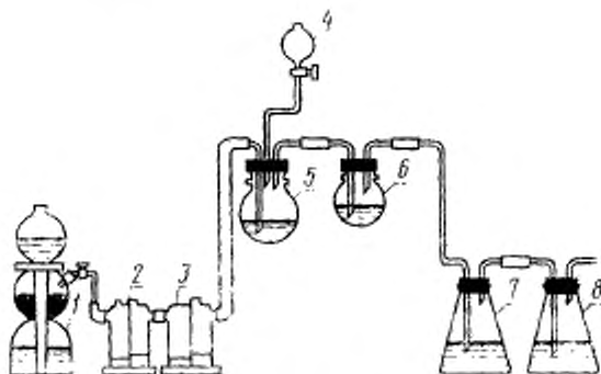
1—аппарат Киппа для получения углекислого газа; 2—склянка Тимченко с раствором сульфата меди; 3—склянка Тимченко с водой; 4—капельная поронка; 5—колба вместимостью 500 см 3 для разложения шпата; 6—колба для улавливания паров соляной кислоты; 7—первый приемник; 8—второй приемник
