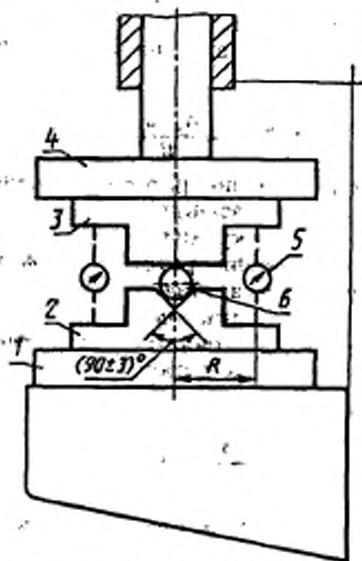
1 и 4 — плиты; 2 и 3 — стальные призмы; 5 — индикатор; 6 — шарик
