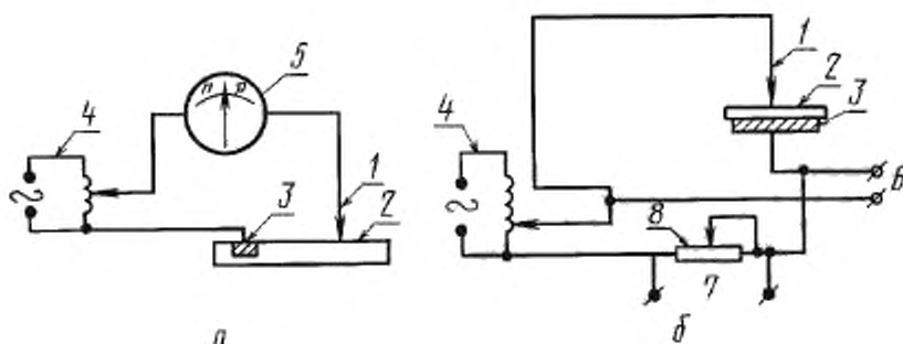
1 — точечный контакт (зонд); 2 — монокристаллический слиток; 3 — омический контакт; 4 — автотрансформатор; 5 — нуль индикатор; 6 — отвод к горизонтальным пластинкам осциллографа; 7 — отвод к вертикальным пластинкам осциллографа; 8 — регулировочное сопротивление
