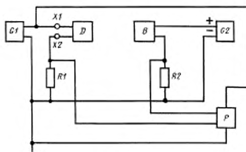
G1 — генератор импульсов тока; R1 — согласующий и тока задающий резистор; X1 , X2 — контакты подключения излучателя, D — излучатель, B — фотоприемник; R2 — резистор нагрузки; G2 — регулируемый генератор постоянного напряжения; P — измеритель временных интервалов (осциллограф)
