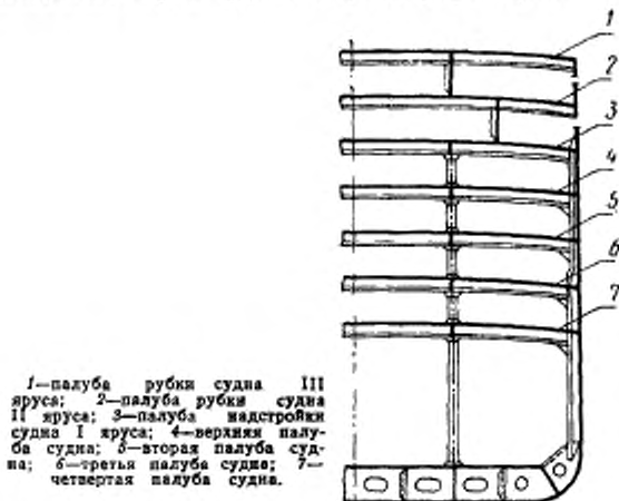
Черт. 1 Схема расположения палуб на судне
