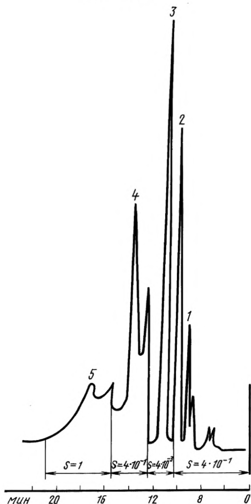
Хроматограмма
