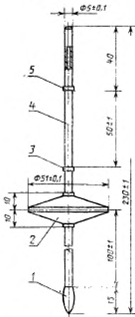
1—труба-наконечник; 2—латунный поплавок; 3 и 5—кольца; 4—стержень
