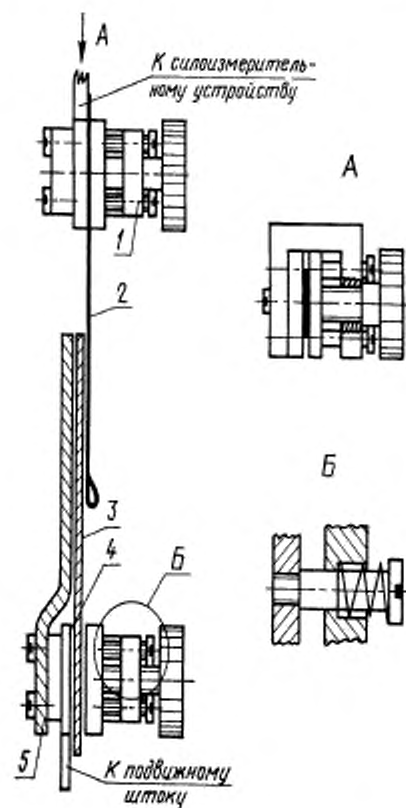
1 — неподвижный зажим; 2 — фольга; 3 — пленка лака (эмали), армированная стеклотканью; 4 — подвижный зажим; 5 — направляющая планка
