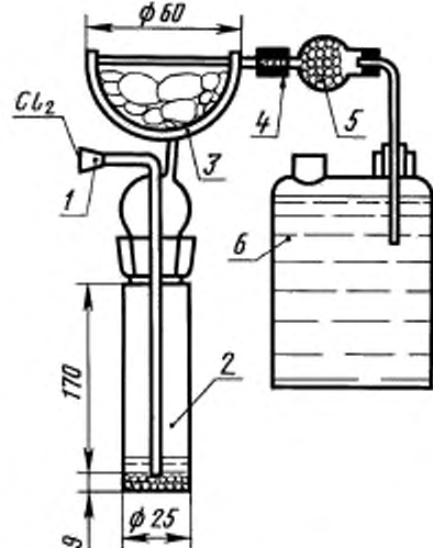
1 — шлиф; 2 — пробирка с навеской олова и четыреххлористым углеродом; 3 — довшка, охлажденная льдом; 4 — трубка резиновая; 5 — трубка с хлористым кальцием; 6 — склянка со щелочью (10 %-ный раствор) для поглощения избытка хлора
