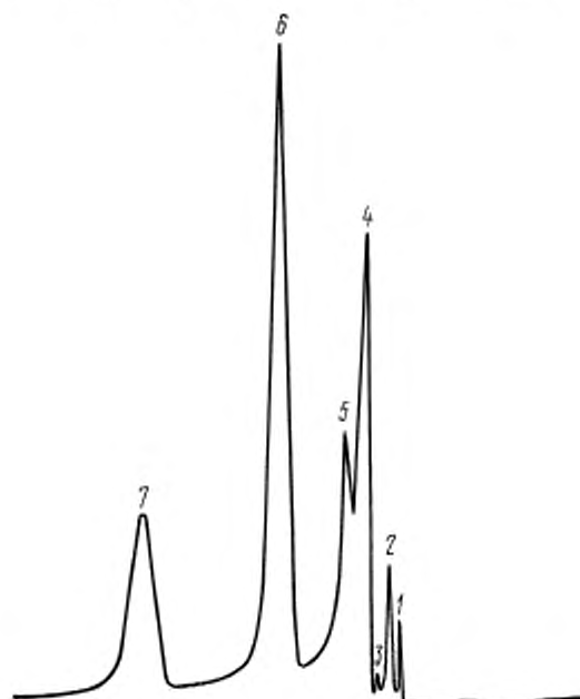
Типовая хроматограмма технической муравьиной кислоты
