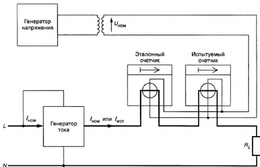
Рисунок А.1 — Схема испытательной цепи (справочная)
