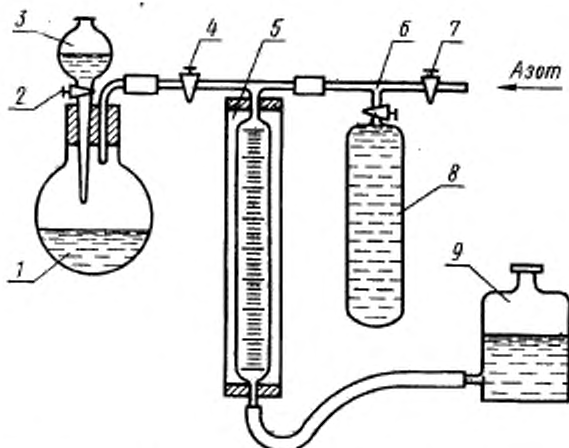
1—реакционная колба вместимостью 25—30 см 3 ; 2, 4, 6, 7—краны; 3—капельная воронка; 5—измерительная бюретка вместимостью 100 см 3 с водяной рубашкой; 8—поглотительная склянка; 9—уровнительный сосуд.
