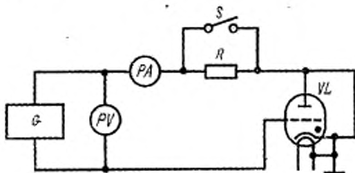
R — резистор; S — выключатель; PV — измеритель напряжения; PA — измеритель тока; VL — испытываемый тиратрон; G — источник постоянного напряжения
