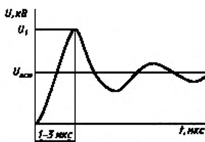
Рисунок Д.2 — Форма грозовых импульсов, характерная для точек присоединения a , b , z , d на рисунке Д.1.
