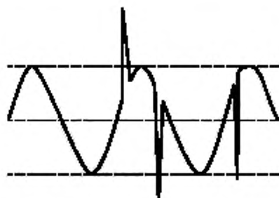
Рисунок А.3 — Импульсы напряжения
