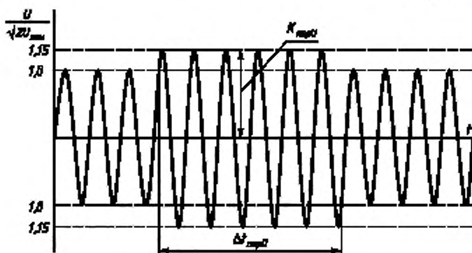
Рисунок Б.4 — Временное перенапряжение
