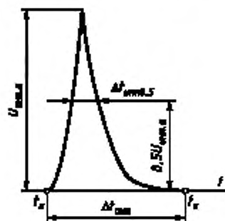
Рисунок Б.3 — Параметры импульсного напряжения
