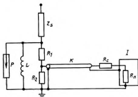
I — измерительный прибор с входным сопротивлением R_i ; K — радиочастотный кабель; P — разрядник; Z_s — элемент связи; L — катушка индуктивности; R_2 — резистор, согласующий вход измерительного прибора с волновым сопротивлением кабеля; R_1 и R_3 — резисторы
